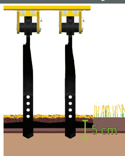
Křídlová radlička: Pracovní hloubka do 5 cm
