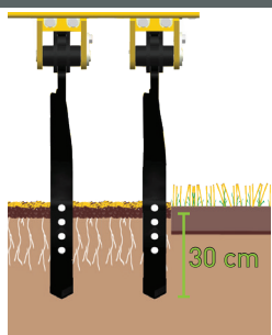
Dlátová radlička: Pracovní hloubka až 30 cm
