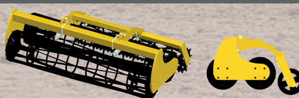
Válec Twin crumbling Ø400 + válec finisher Ø320
