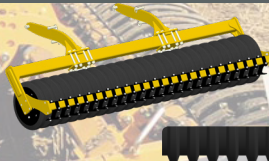
Prútvý valec Ø526 + Finisher Ø460
