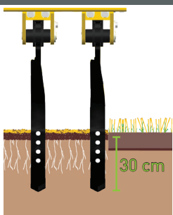
Dlátová radlička: Pracovná hĺbka až 30 cm
