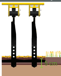
Krídlová radlička: Pracovná hĺbka do 5 cm
