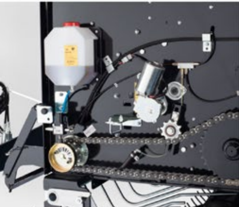
Automatické mazání hnacího řetězu Automatické mazanie hnacej reťaze Automatische Schmierung von Ketten Automatyczne smarowanie łańcuchów Автоматическая смазка цепей
